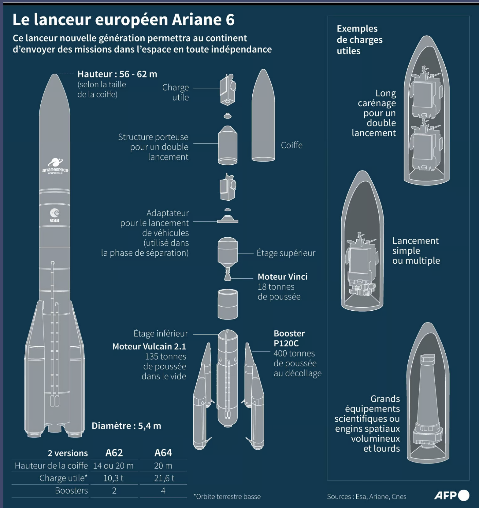
Figure 1. Illustration d'Ariane 6, la nouveau lanceur européen
